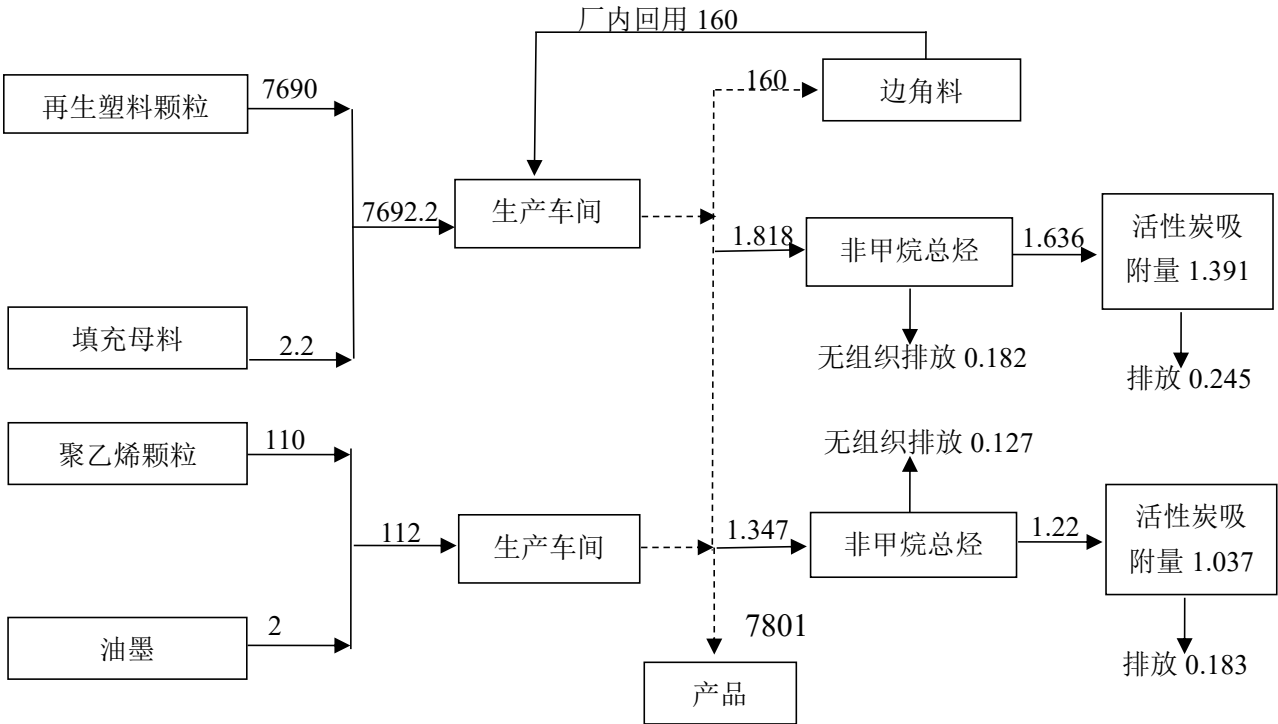
图 3.2-2 项目物料平衡图 单位：t/a
