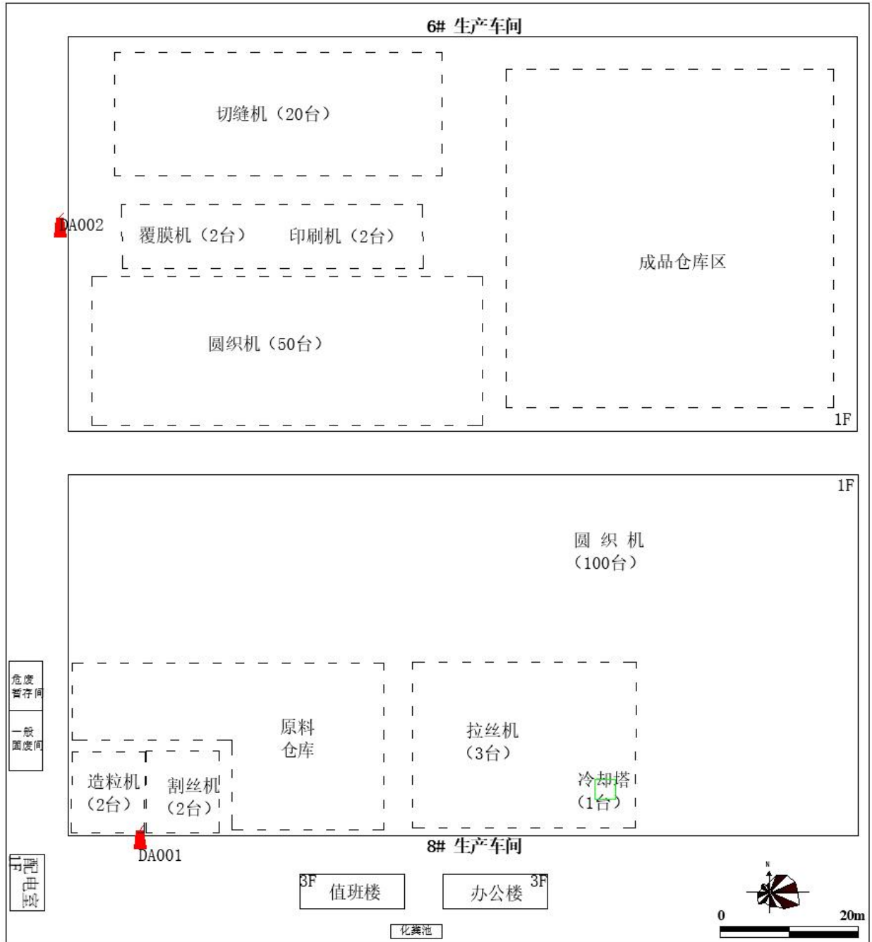
图 3.1-1 变更前总平面布置图
