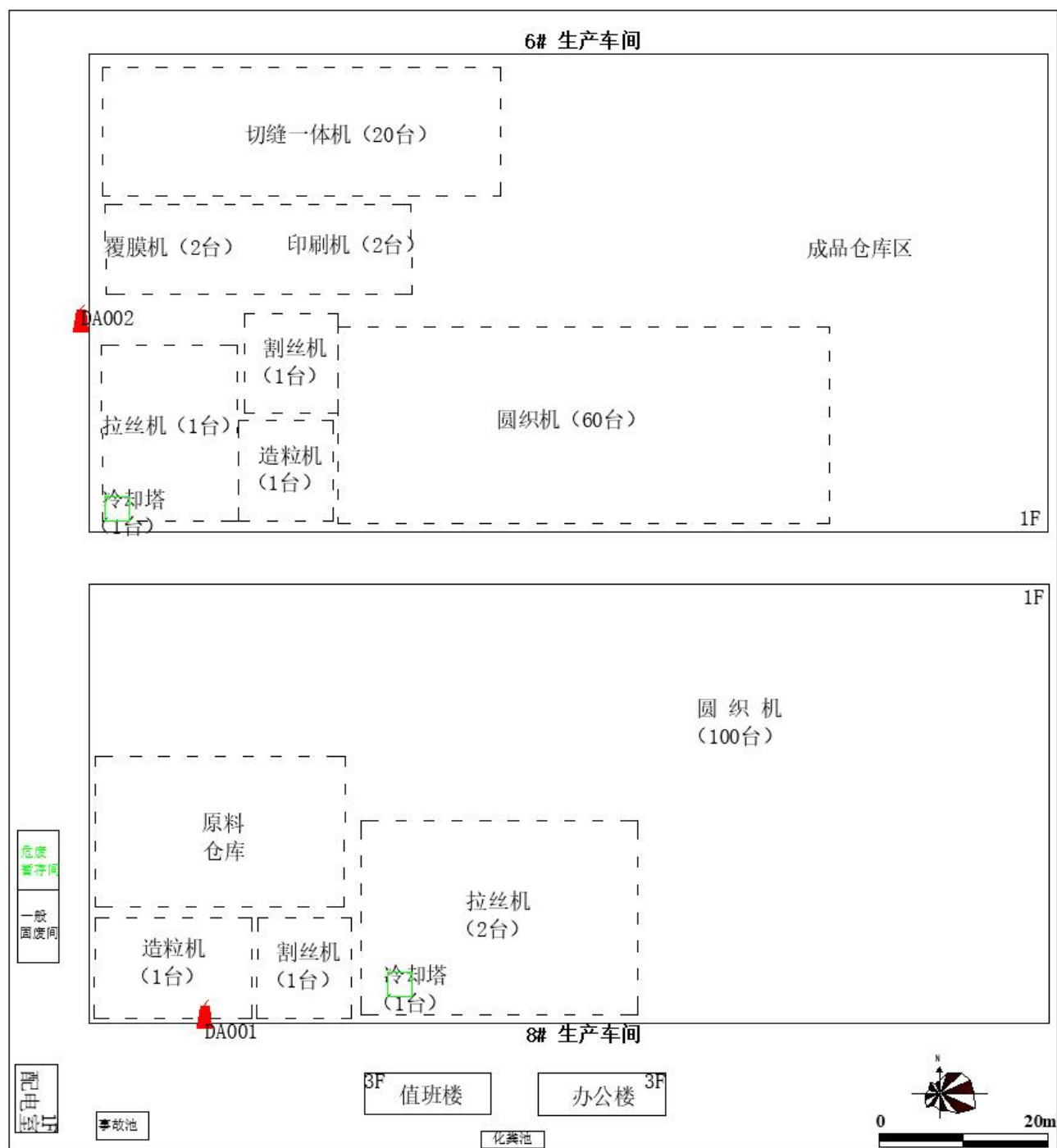
图 3.1-2 变更后总平面布置图
